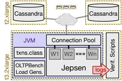
Fig. 21. Testing framework
